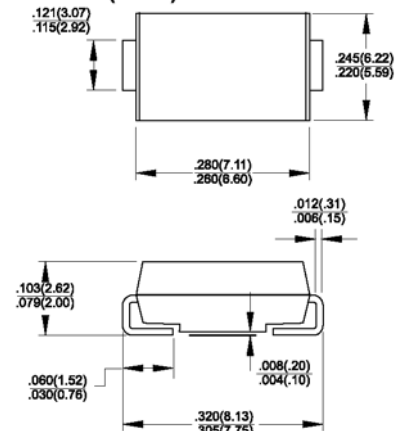
DO-214AB (SMC)
